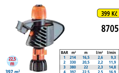
postřikovač - TURBOSPIKE
